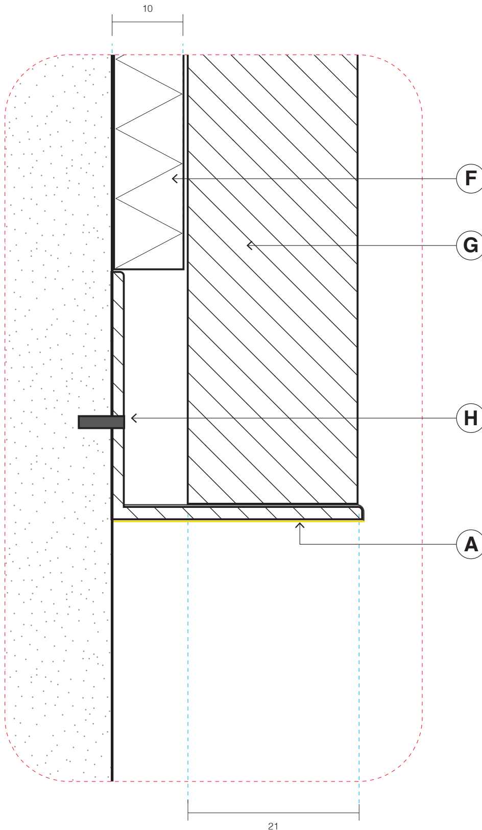
02 Detail Bottom edge Scale 2:1
